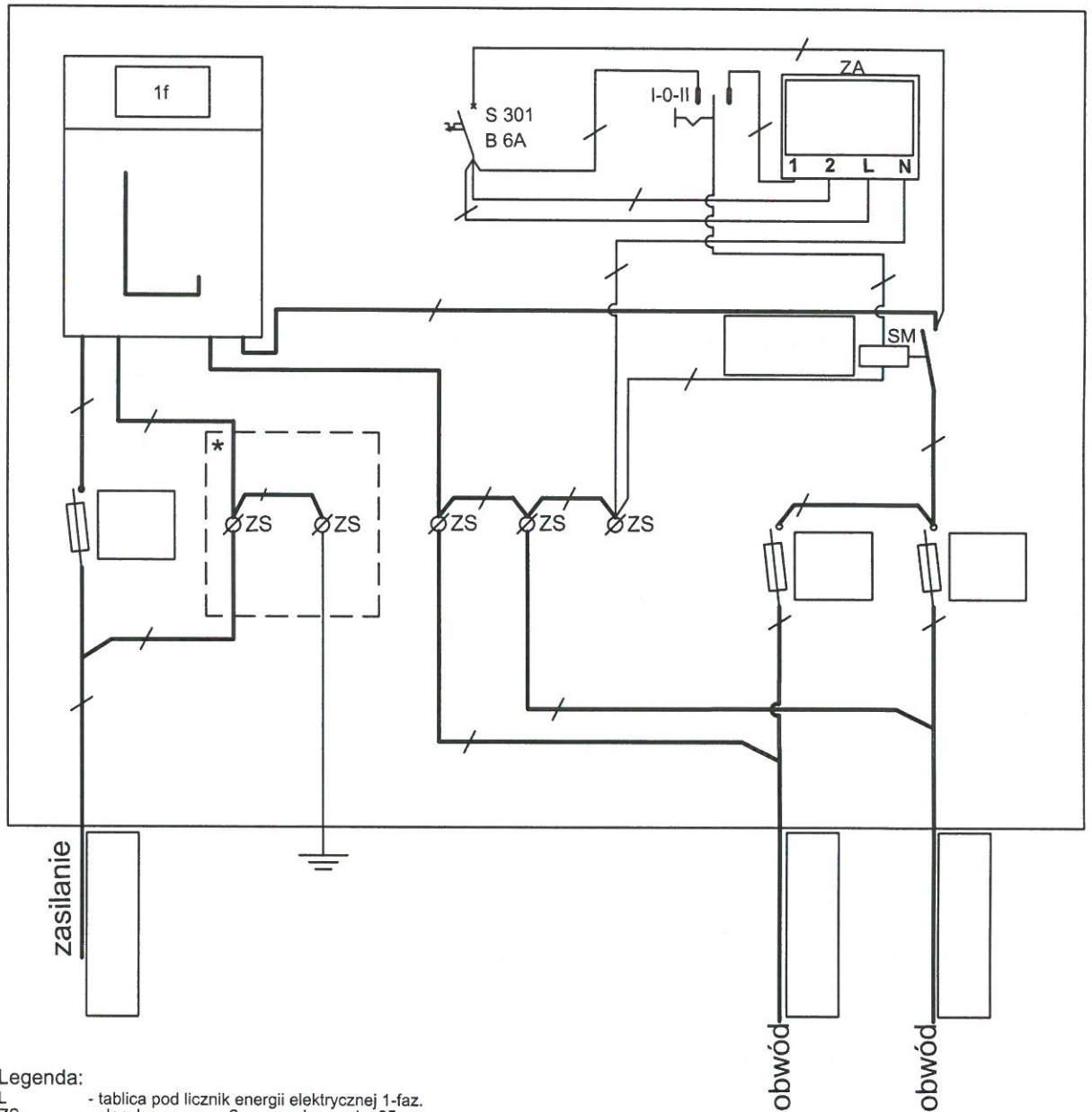
Schemat szafki oświetleniowej pomiarowo-sterującej 1-fazowej, z obwodami 2x 1-faz.
